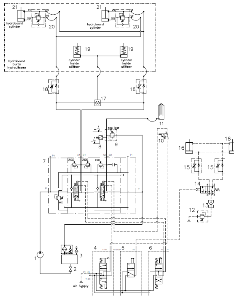
7.16. Schemat hydrauliczny wywrotki trójstronnej z zaworem pneum. żuraw/wywrotka
