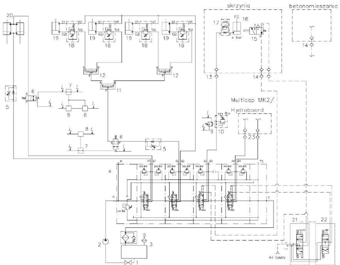
7.12. Schemat hydrauliczny wywrotki trójstronnej z instalacją 2ob. 4 przew. zestawienie części
