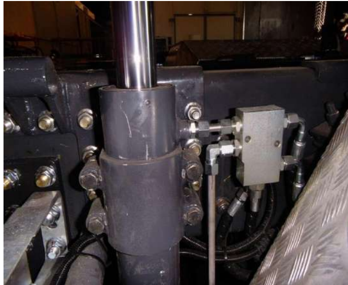
Rys. 50. Siłownik podnoszenia/opuszczania
