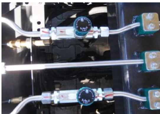
Rys. 16. Zawory dławiące burty hydraulicznej
