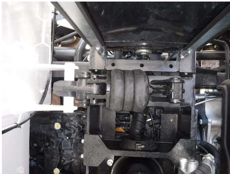
f) Rahmenbefestigungen
